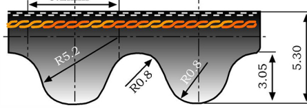
S8M Zaman Kayışları
