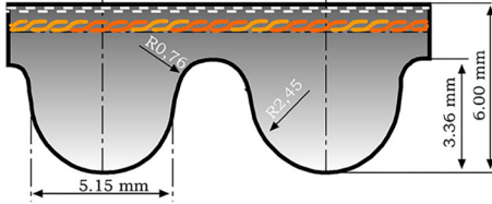
HDT 8M Zaman Kayışları
