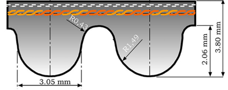
HDT 5M Zaman Kayışları
